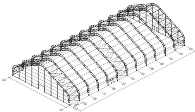
СХЕМА АНГАРА тип Д
