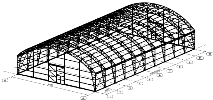
СХЕМА АНГАРА тип В
