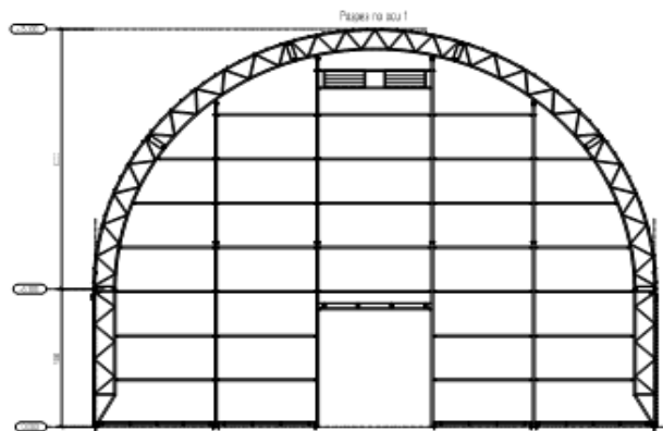
СХЕМА АНГАРА тип В
