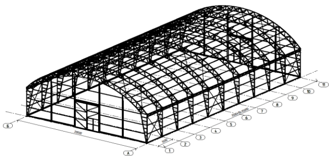
СХЕМА АНГАРА тип В
